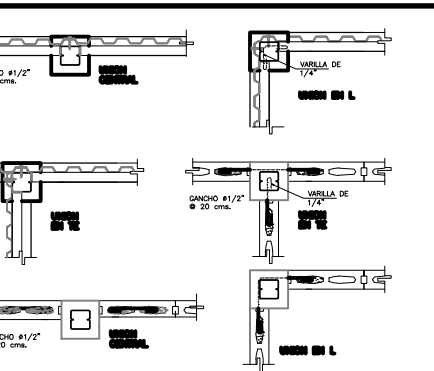
DETALLES DE UNIONES esc. 1:12.5
