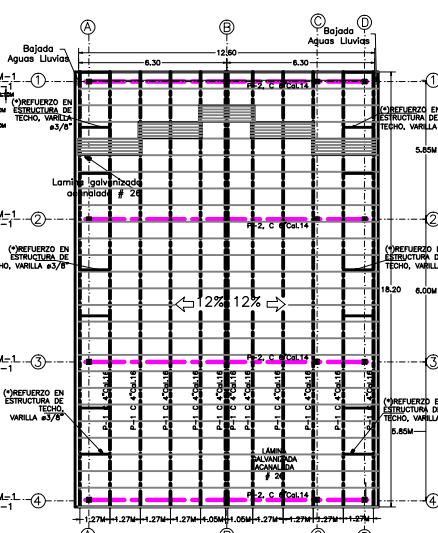
PLANTA ESTRUCTURAL DE TECHOS esc. 1:100
