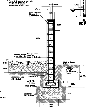
DETALLE DE COLUMANA DONDE HAY PARED DE BLOQUE
