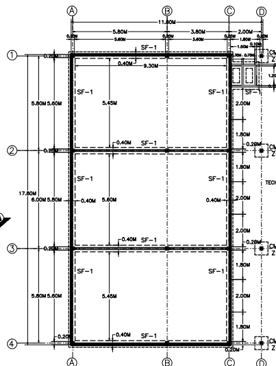
PLANTA DE FUNDACIONES esc. 1:100
