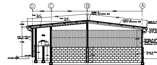
SECCION A - A esc. 1:75
