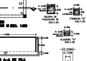
SOLERA DE FUNDACION esc. 1:20
