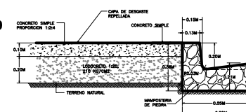
SOLERA DE FUNDACION esc. 1:20
