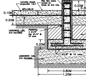
SOLERA DE FUNDACION esc. 1:20
