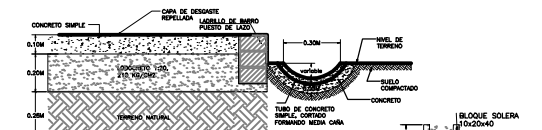
DETALLE DE PISO TIPO ACERA Y CANALETA DE AGUAS LLUVIAS esc. 1:10
