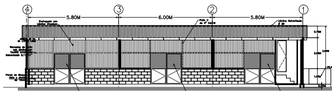
ELEVACION PRINCIPAL esc. 1:75
