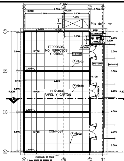
PLANTA ARQUITECTONICA esc. 1:100
