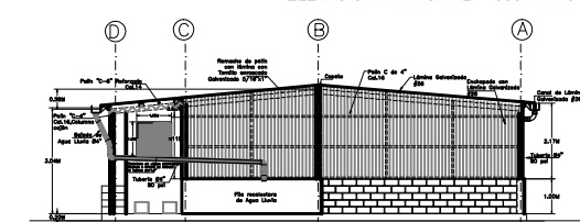
ELEVACION LATERAL esc. 1:75
